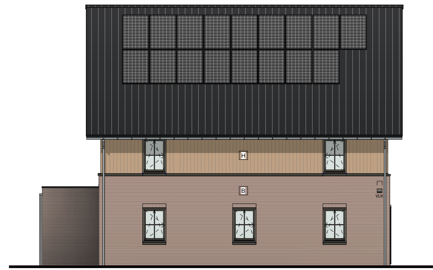
Linker zijgevel
