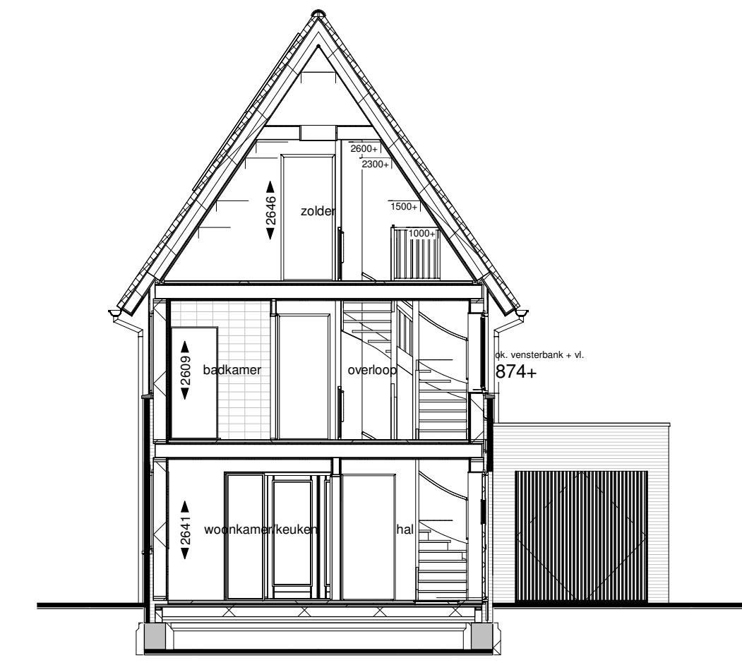
Doorsnede B
