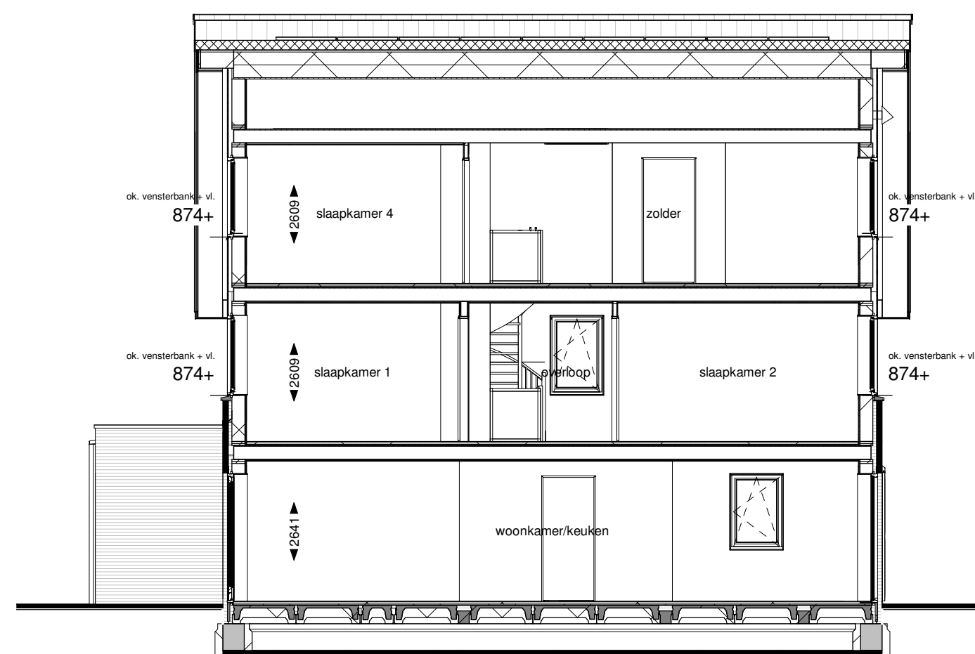
Doorsnede A
