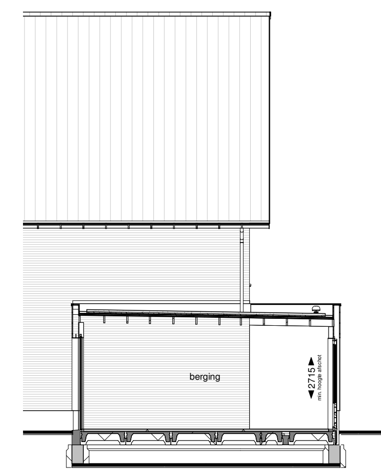
Doorsnede C
