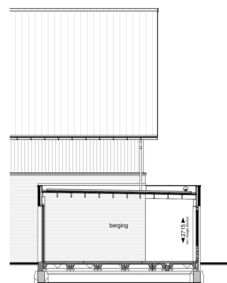
Doorsnede C
