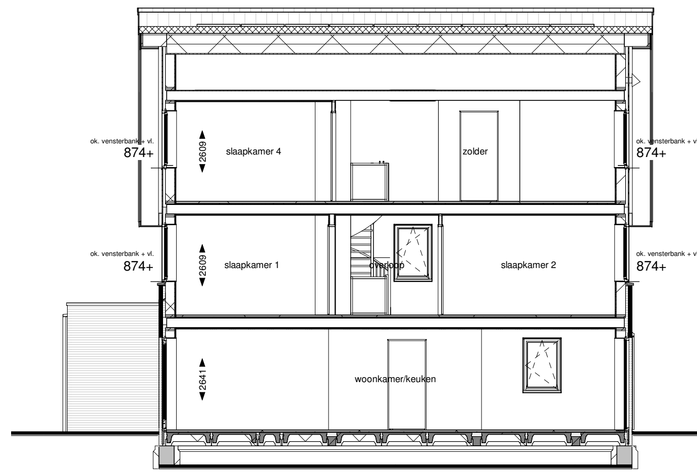
Doorsnede A
