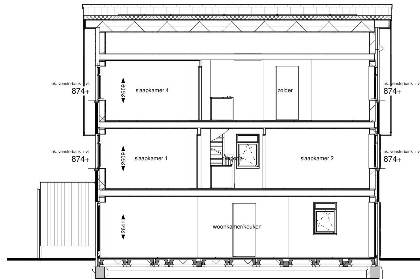
Doorsnede A
