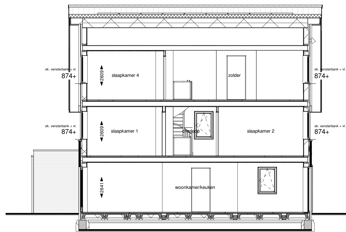
Doorsnede A
