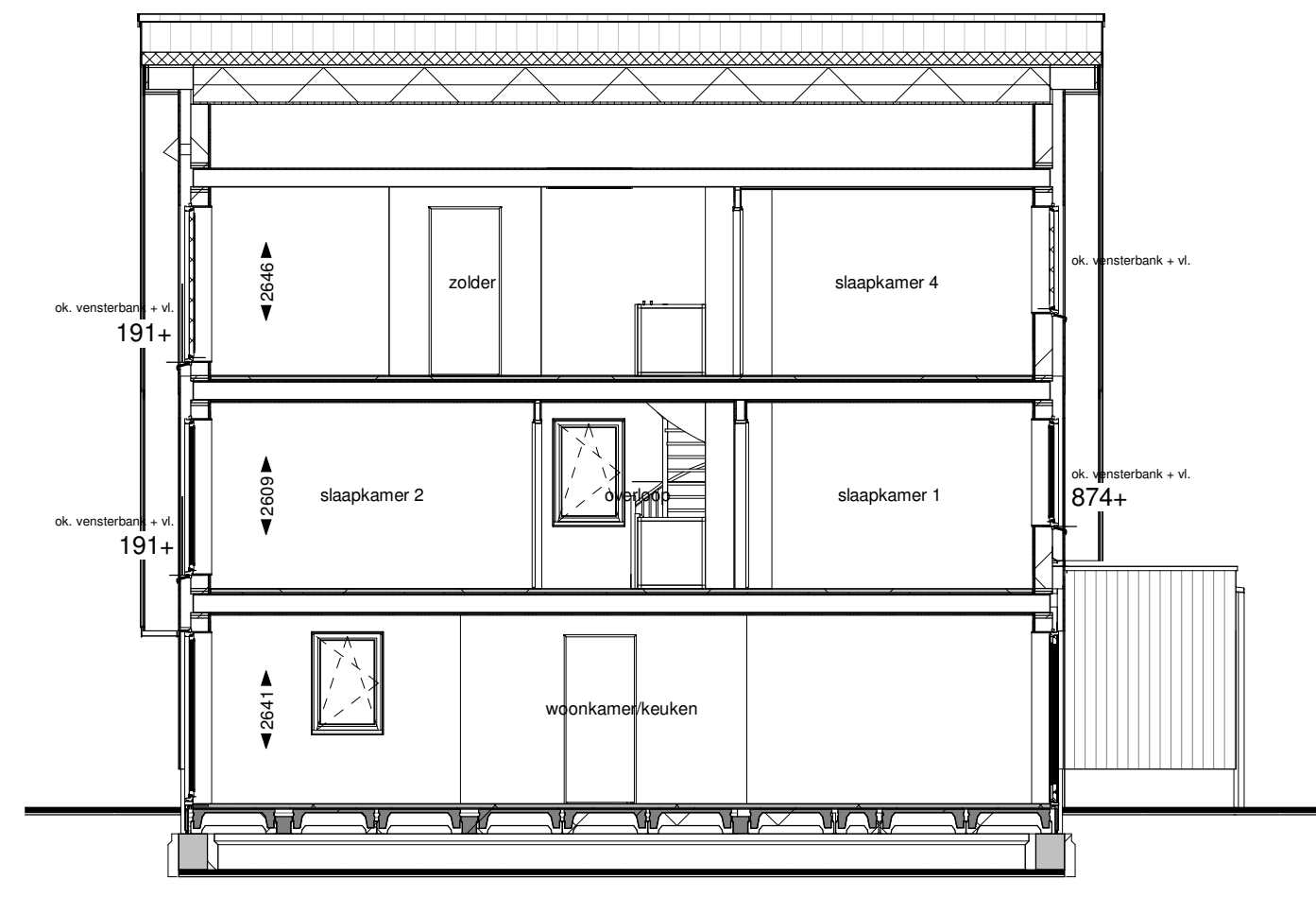
Doorsnede A
