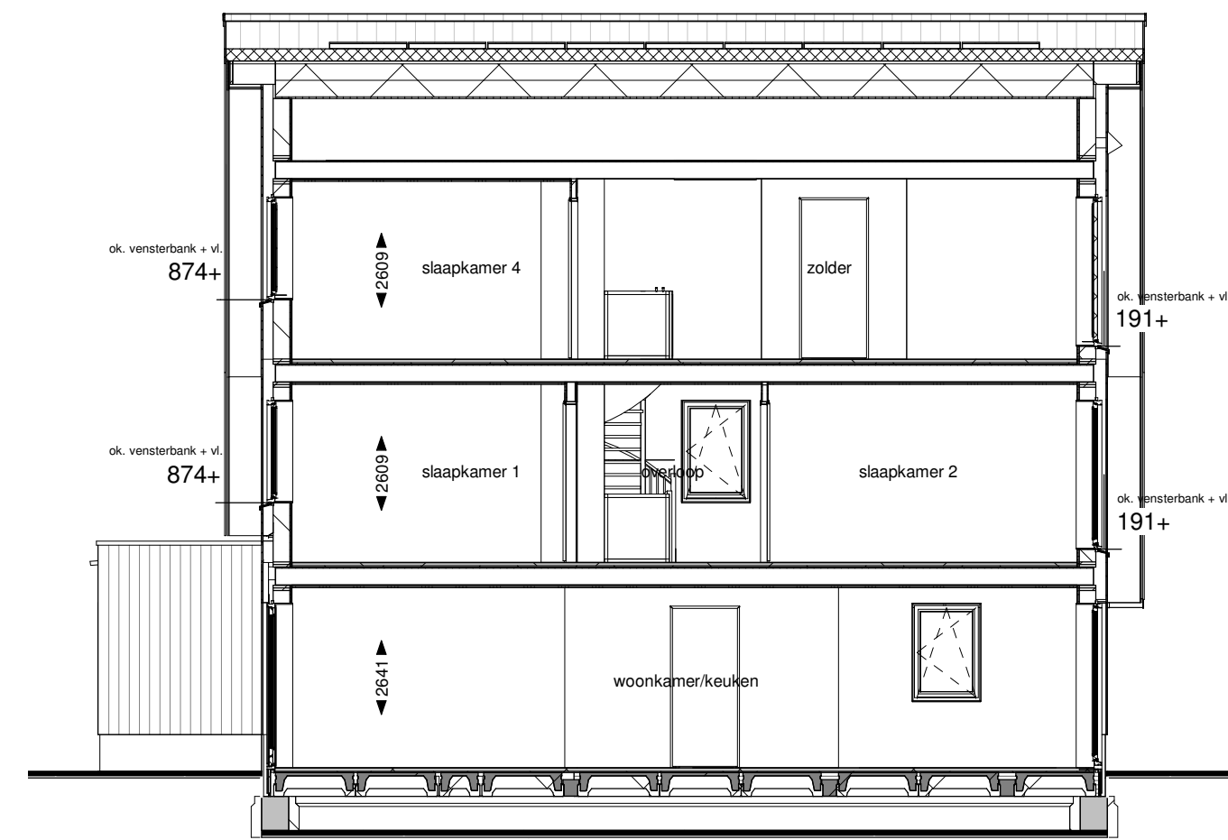
Doorsnede A
