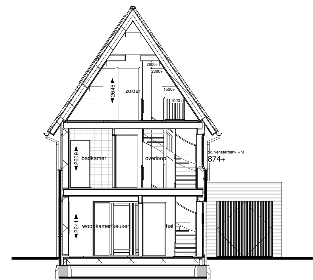
Doorsnede B
