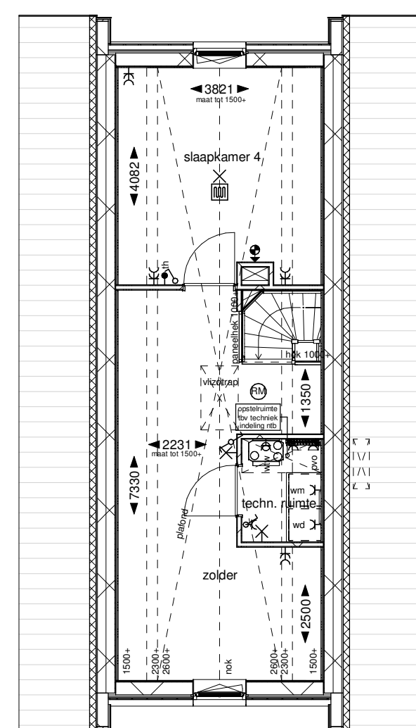
Tweede verdieping
