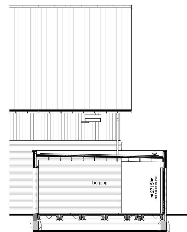
Doorsnede C
