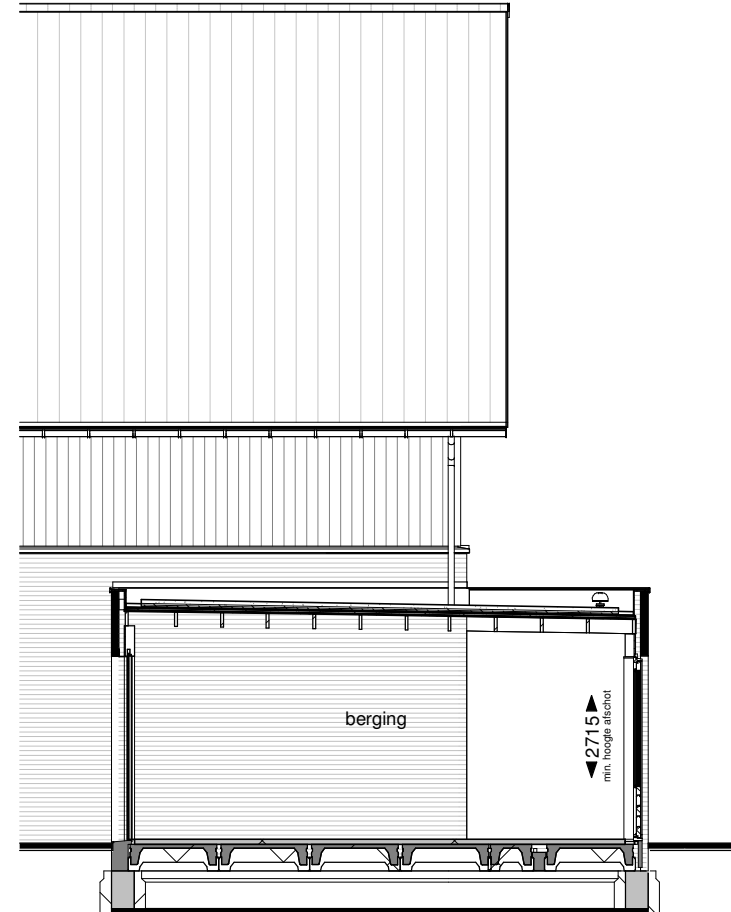
Doorsnede C
