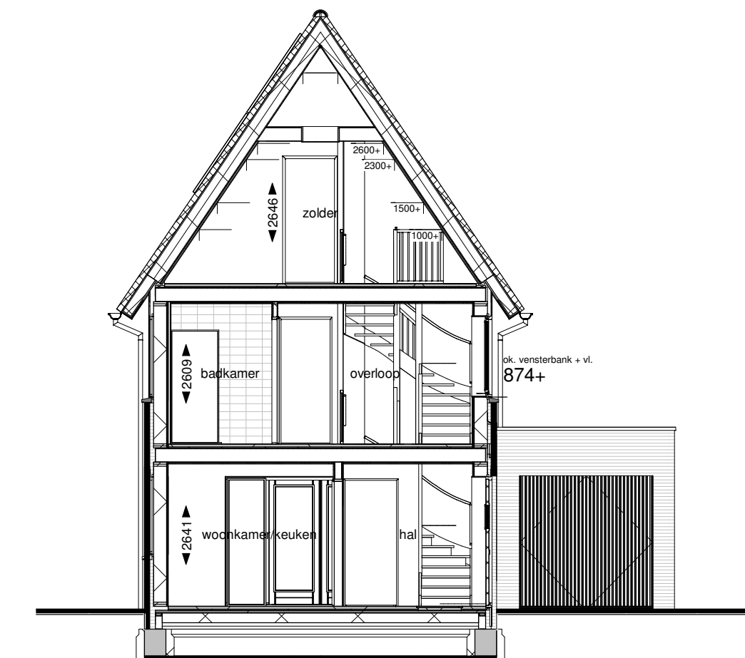
Doorsnede B
