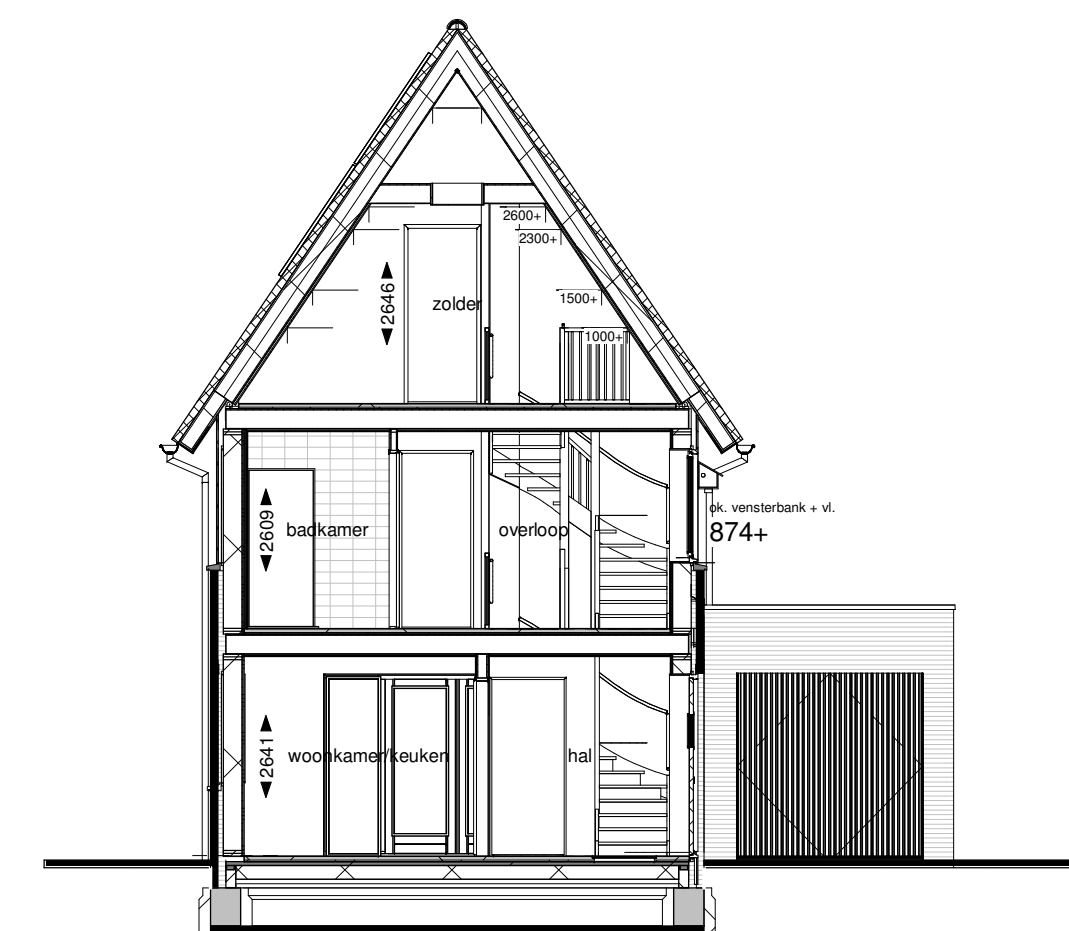
Doorsnede B
