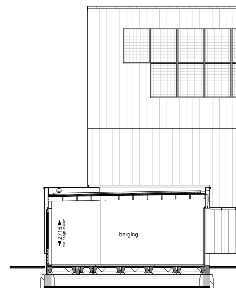
Doorsnede C
