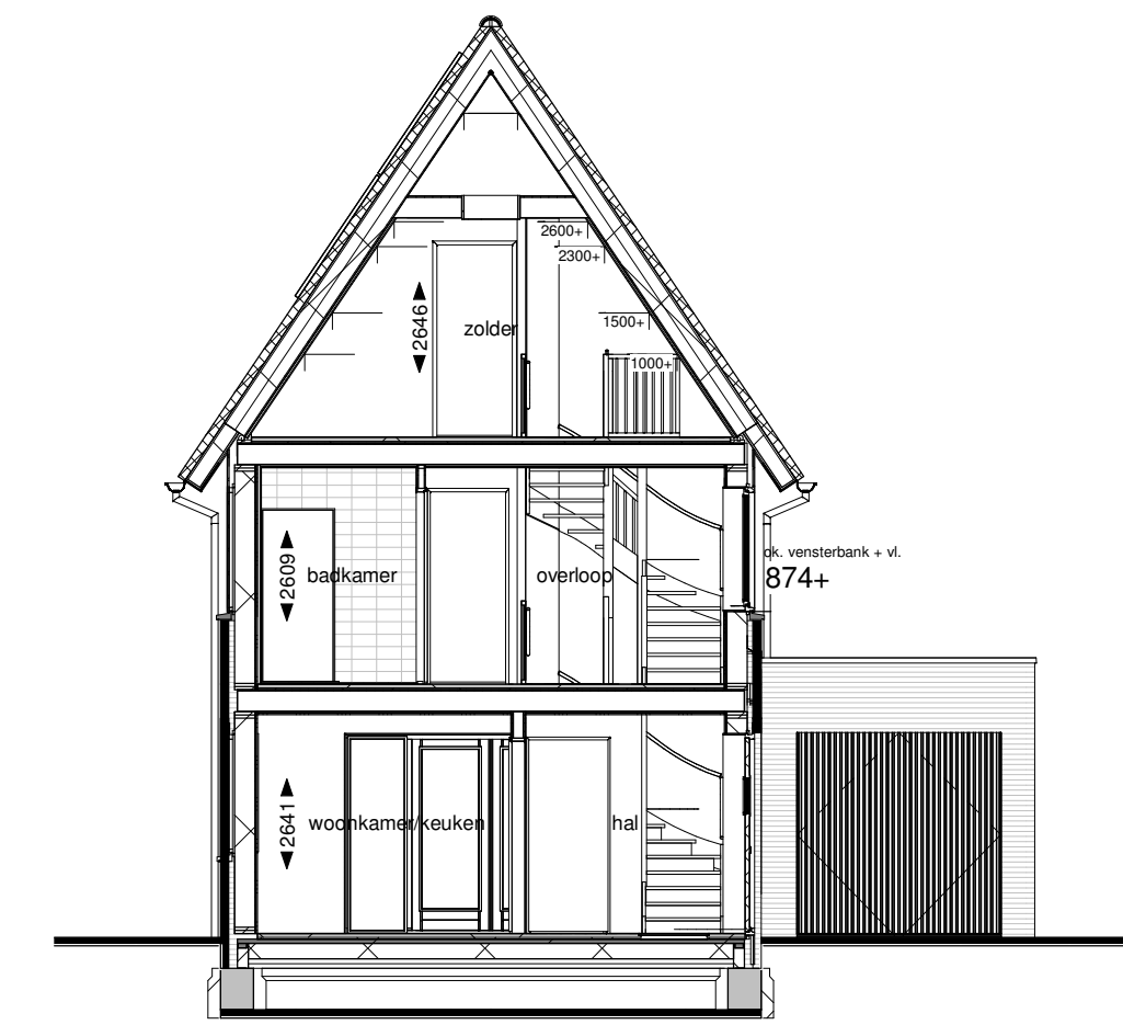
Doorsnede B
