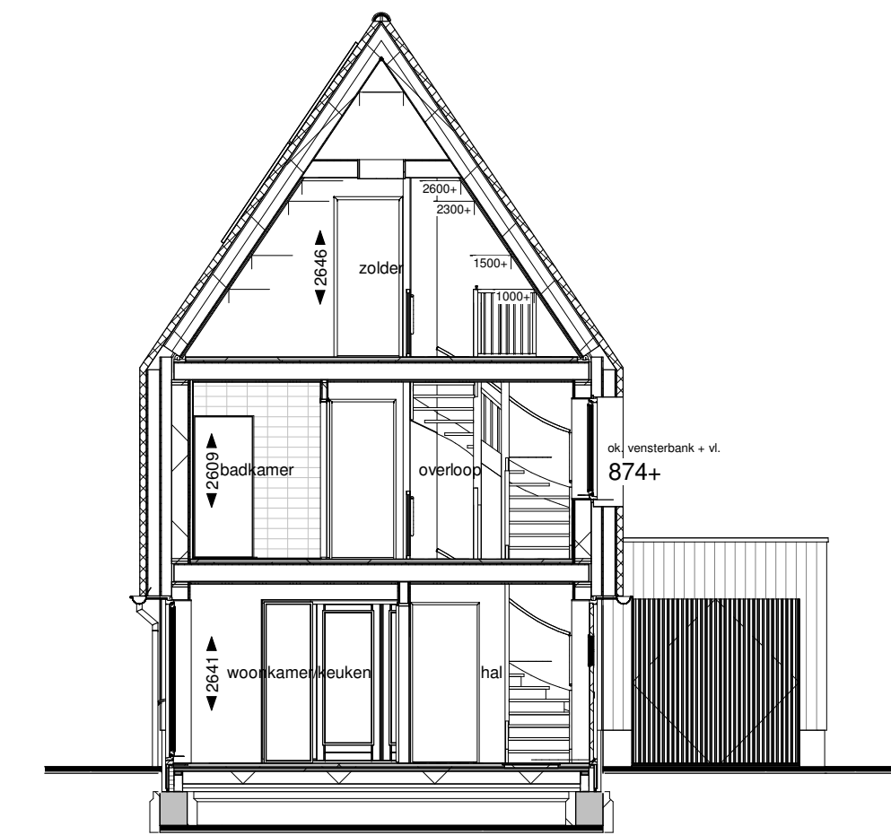
Doorsnede B
