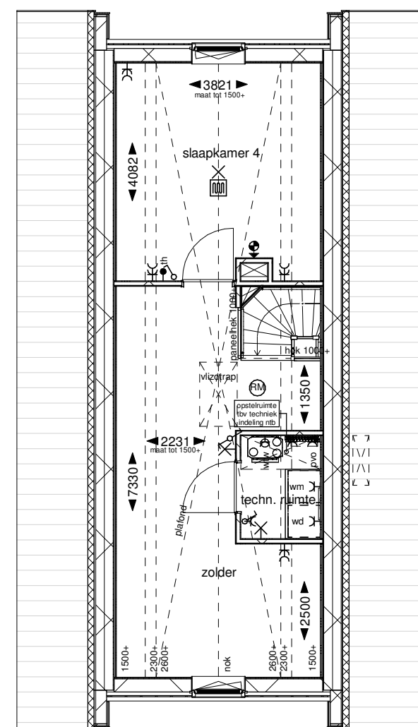
Tweede verdieping
