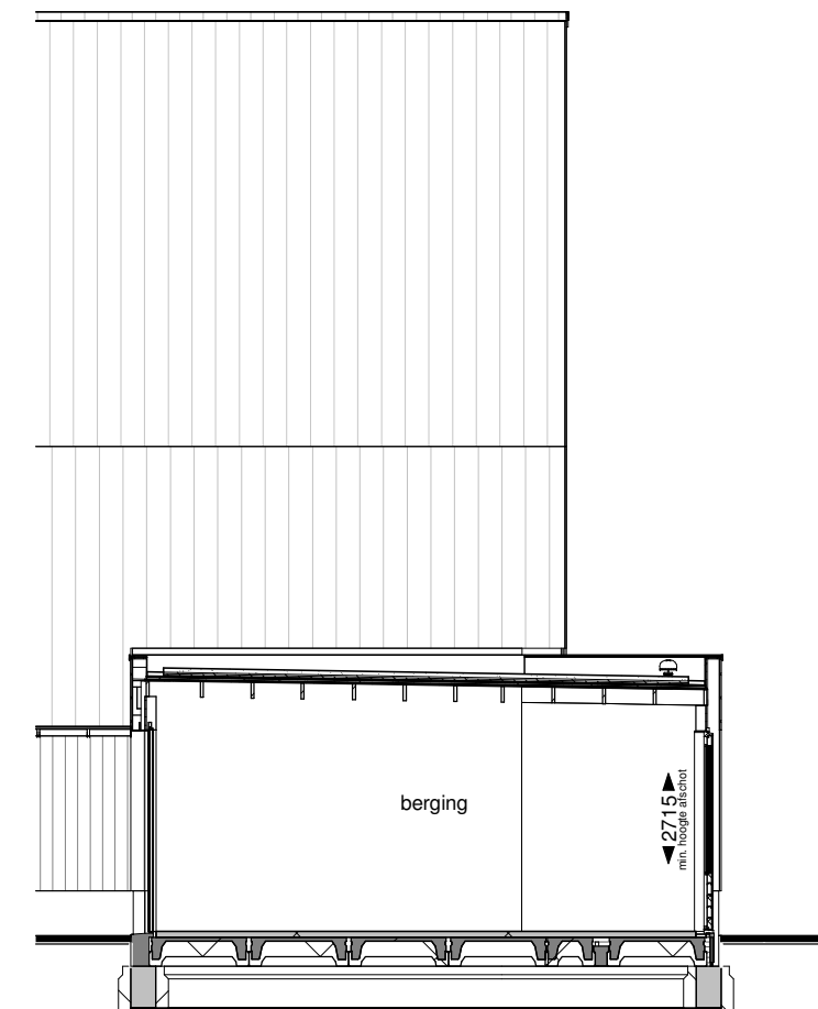
Doorsnede C
