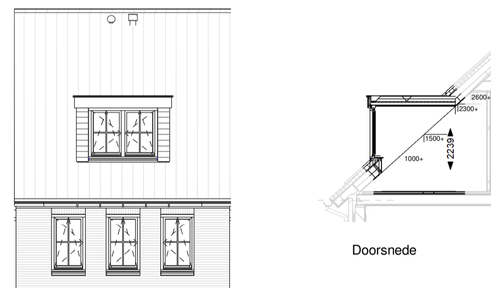
Voorgevel
