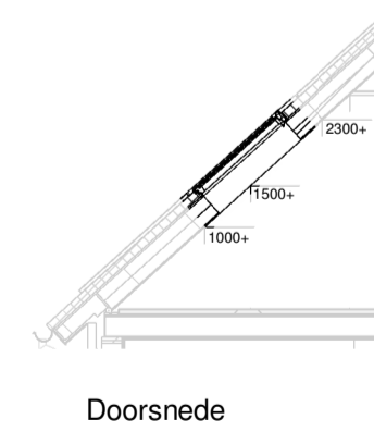
Doorsnede
