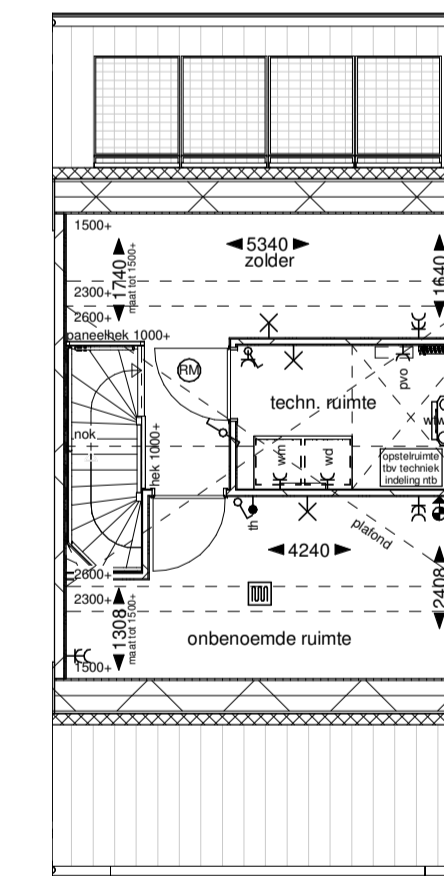
Tweede verdieping
