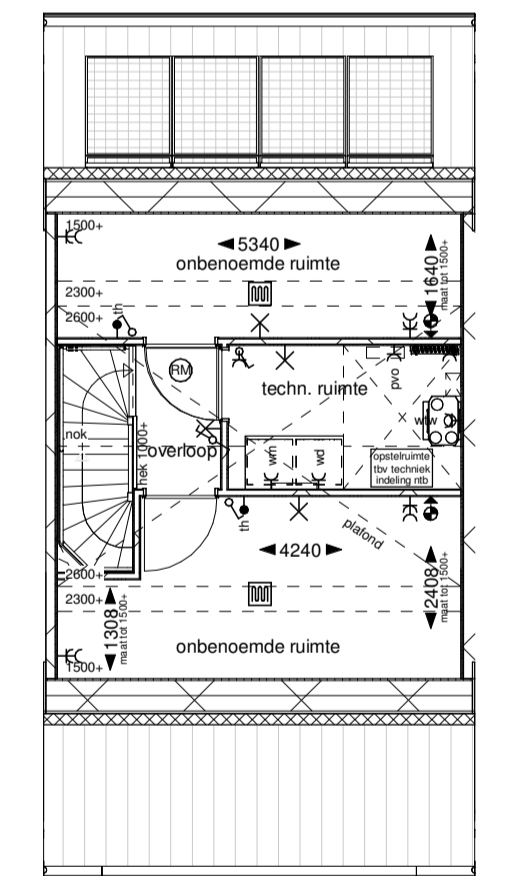
Tweede verdieping
