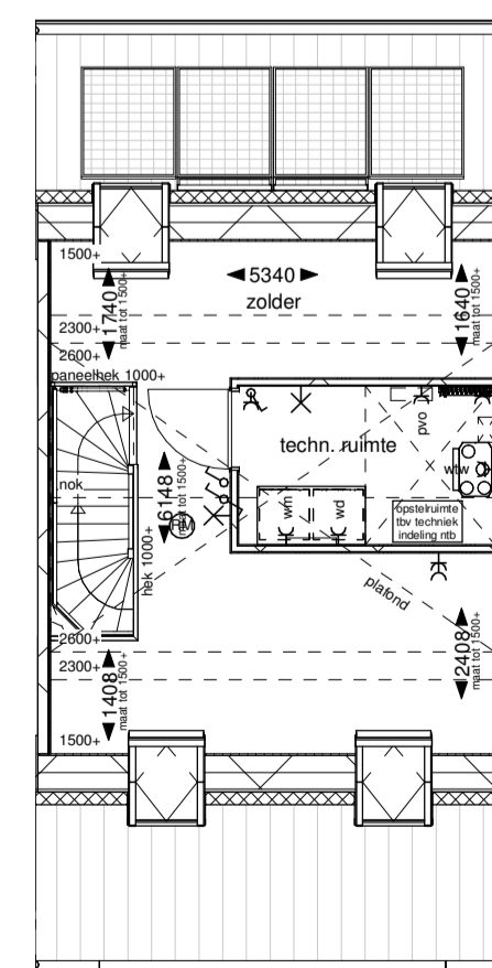
Tweede verdieping
