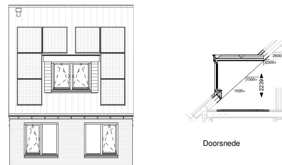
Achtergevel
